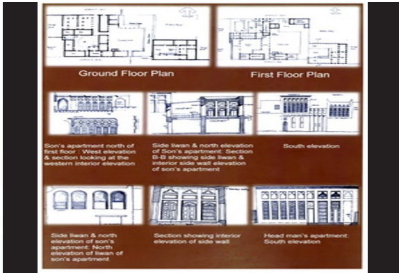
الفائز بالجائزة الثالثة (مناصفة) عن بحث (ترميم منزل فخرو «بيت التجار»)، مجموعة طالبات من جامعة البحرين - كلية الهندسة - مملكة البحرين
