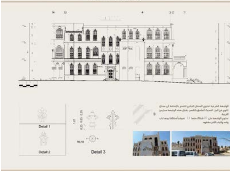
توثيق الواجهة الشرقية
