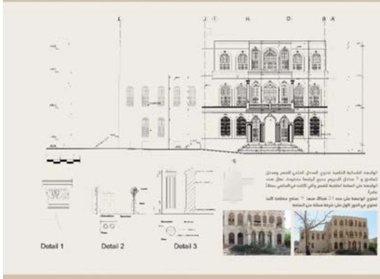
توثيق الواجهة الشمالية
